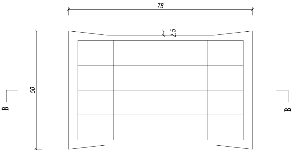
盖板钢筋平面布置图
