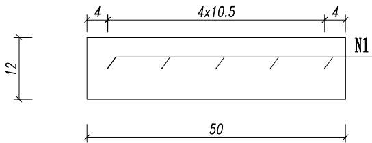
A-A
