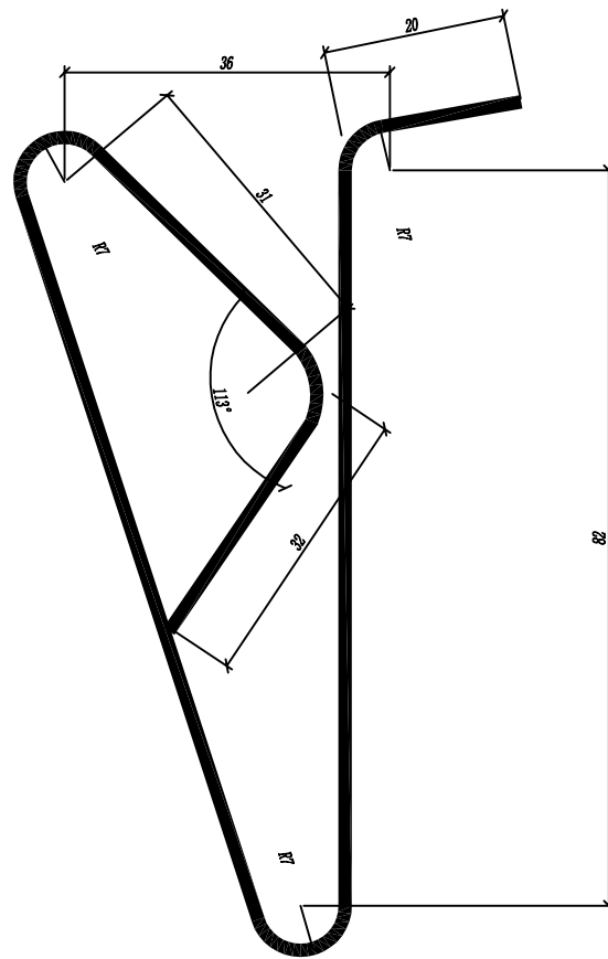
吸音板卡簧(180x30x1.6)
