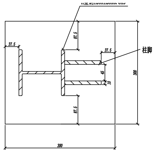
上法兰板
