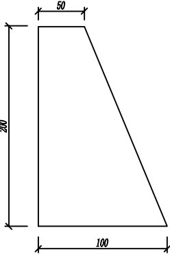
柱脚 厚10t
